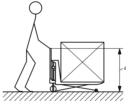
Figure 5 — Tiller (pulling)
